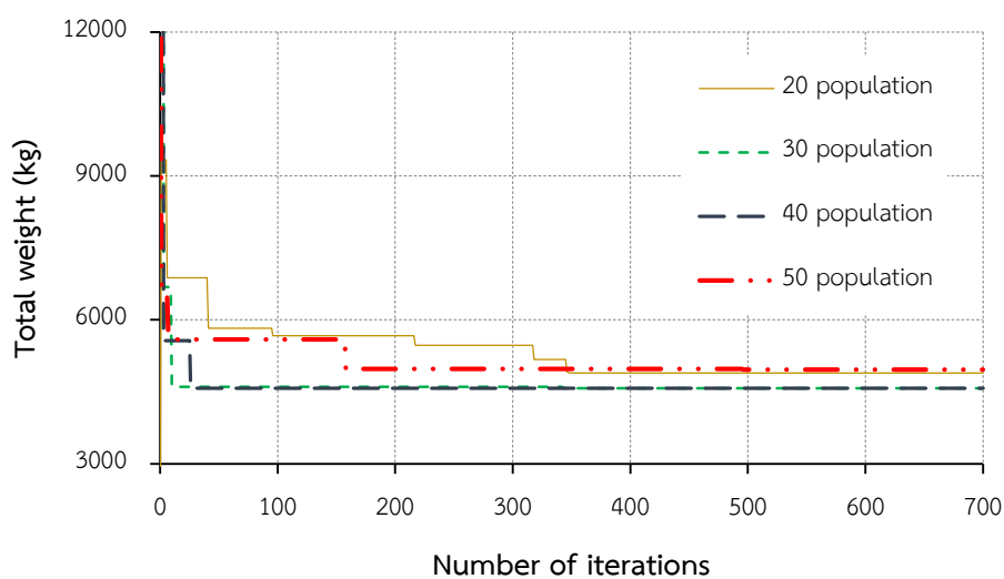
ภาพประกอบ 32 ลักษณะของการลู่ออกค่าคำตอบที่เหมาะสมของ GWO สำหรับตัวอย่างที่ 3 โครงข้อหมุน 10 ชิ้นส่วน โดยใช้หน้าตัดท่อสี่เหลี่ยม
