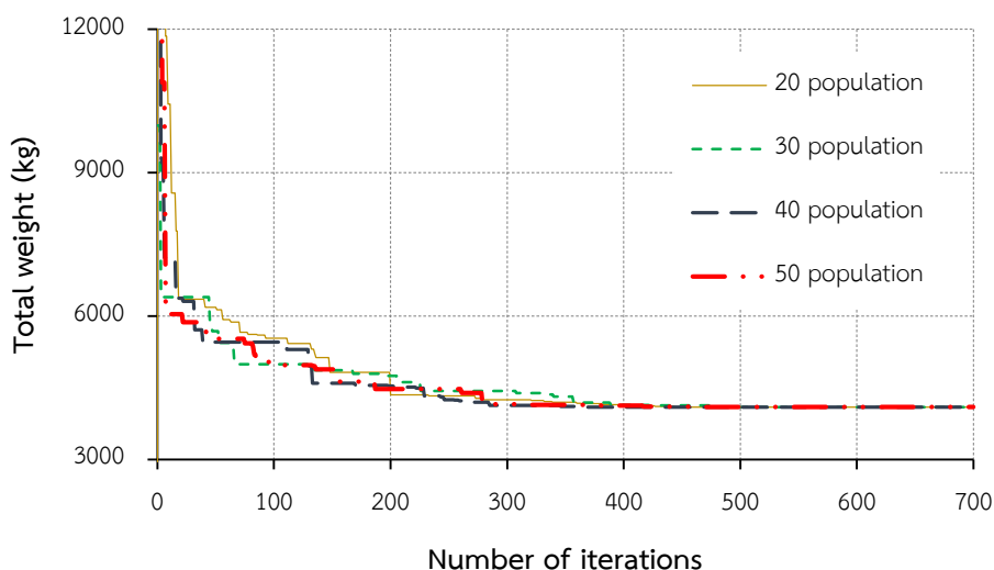
ภาพประกอบ 24 ลักษณะของการลู่เข้าหาคำตอบที่เหมาะสมของ CSA สำหรับตัวอย่างที่ 3 โครงข้อหมุน 10 ชิ้นส่วน โดยใช้หน้าตัดท่อสี่เหลี่ยม
