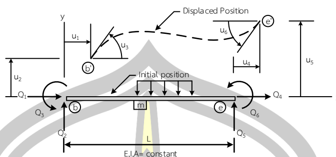
ภาพประกอบ 2 แรงภายในและระยะเคลื่อนที่ของชิ้นส่วนโครงข้อแข็งในระนาบ 2 มิติ
