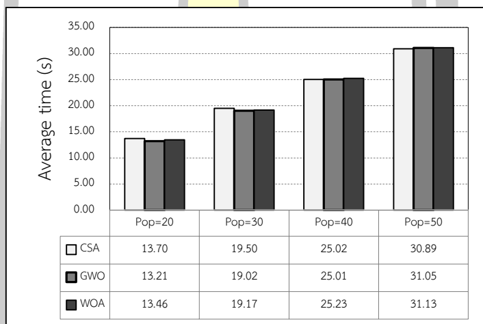
ภาพประกอบ 55 แผนภูมิเวลาเฉลี่ยที่ใช้ในการออกแบบที่เหมาะสมในแต่ละอัลกอริทึมสำหรับ ตัวอย่างที่ 4 สำหรับหน้าตัดท่อนสี่เหลี่ยม
