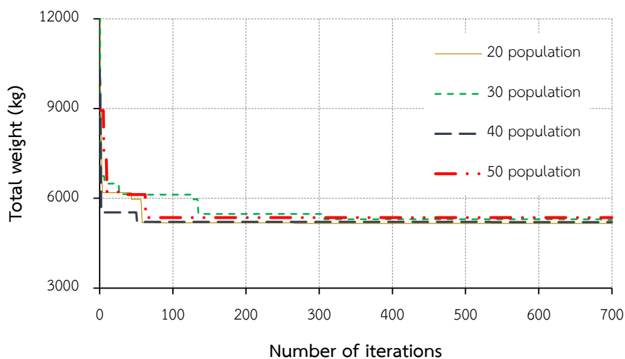
ภาพประกอบ 35 ลักษณะของการลู่เข้าหาคำตอบที่เหมาะสมของ GWO สำหรับตัวอย่างที่ 4 โครงข้อหมุน 18 ชิ้นส่วน โดยใช้หน้าตัดท่อสี่เหลี่ยม
