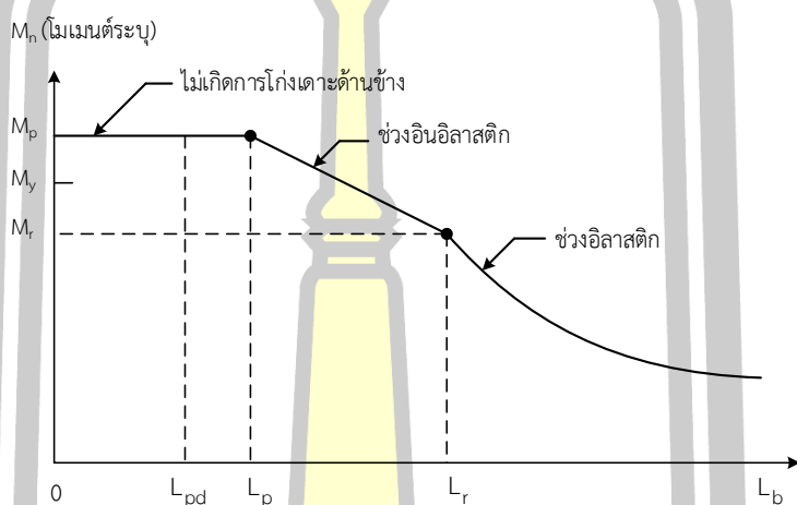
ภาพประกอบ 4 ความสัมพันธ์ระหว่างกำลังแรงดัดระบุกับความยาวปราศจากการค้ำยันด้านข้าง
