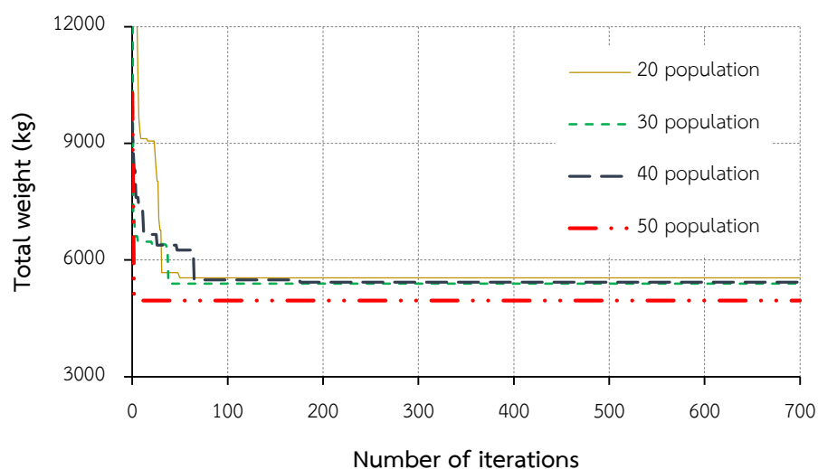
ภาพประกอบ 43 ลักษณะของการลู่เข้าหาคำตอบที่เหมาะสมของ WOA สำหรับตัวอย่างที่ 4 โครงสร้างหมุน 18 ชิ้นส่วน โดยใช้หน้าตัดท่อสี่เหลี่ยม
