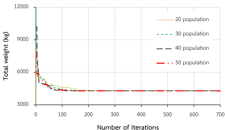
ภาพประกอบ 25 ลักษณะของการลู่เข้าหาคำตอบที่เหมาะสมของ CSA สำหรับตัวอย่างที่ 3 โครงข้อหมุน 10 ชิ้นส่วน โดยใช้หน้าตัดทอกลม
