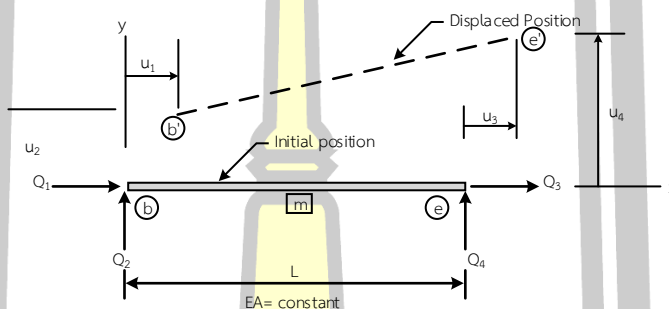
ภาพประกอบ 1 แรงภายในและระยะเคลื่อนที่ของชิ้นส่วนโครงข้อหมุนในระนาบ 2 มิติ
