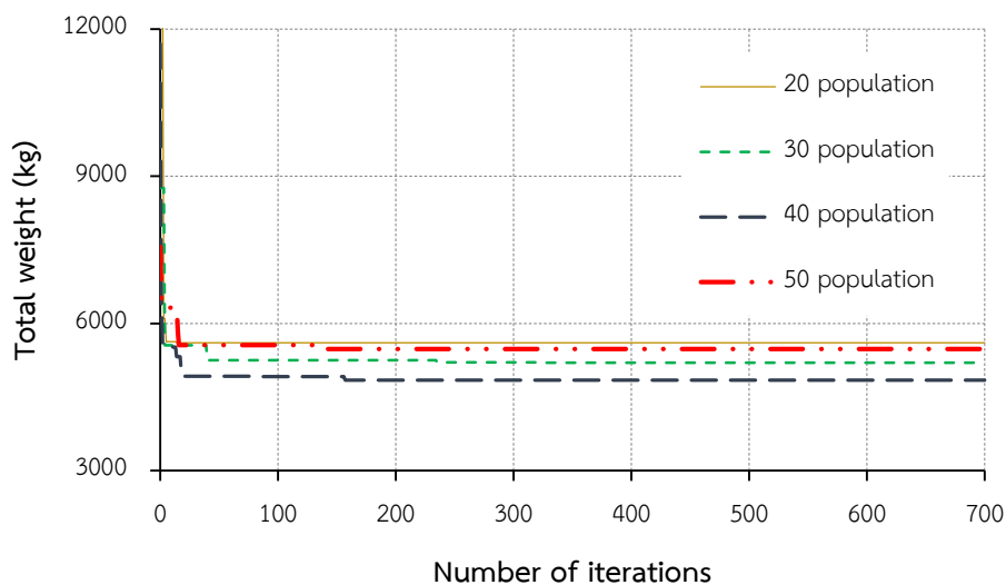
ภาพประกอบ 36 ลักษณะของการลู่ออกหาคำตอบที่เหมาะสมของ GWO สำหรับตัวอย่างที่ 4 โครงข้อหมุน 18 ชิ้นส่วน โดยใช้หน้าตัดท่อกลม
