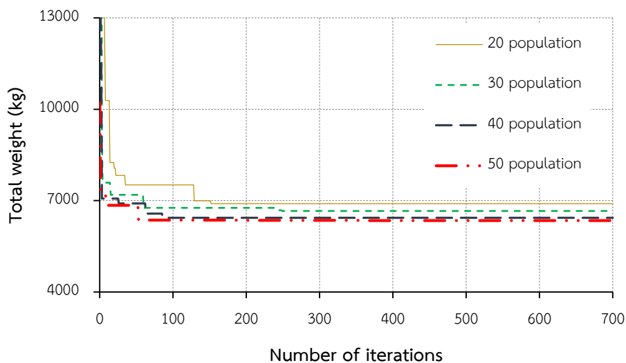
ภาพประกอบ 37 ลักษณะของการลูเข้าหาคำตอบที่เหมาะสมของ GWO สำหรับตัวอย่างที่ 4 โครงข้อ หมุน 18 ชิ้นส่วน โดยใช้หน้าตัดปีกกว้าง
