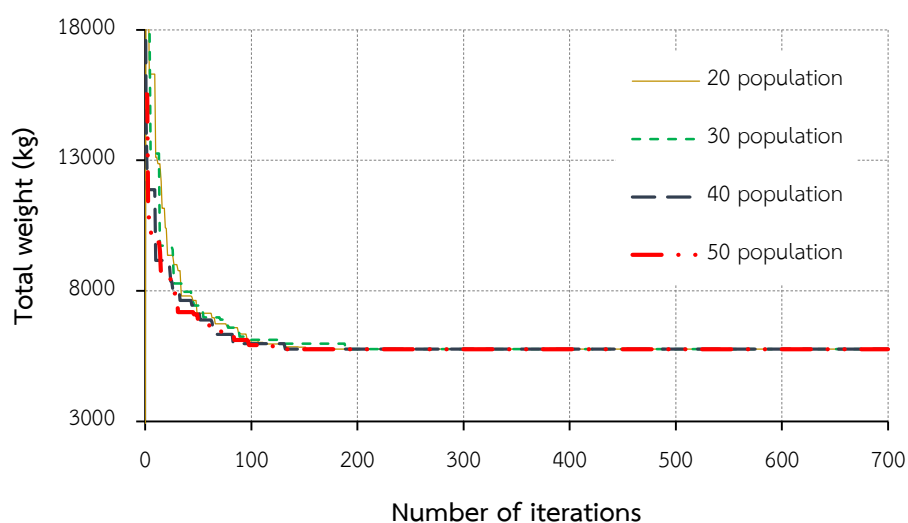
ภาพประกอบ 29 ลักษณะของการหาคำตอบที่เหมาะสมของ CSA สำหรับตัวอย่างที่ 4 โครงข้อ หมุน 18 ชิ้นส่วน โดยใช้หน้าตัดท่อกลม
