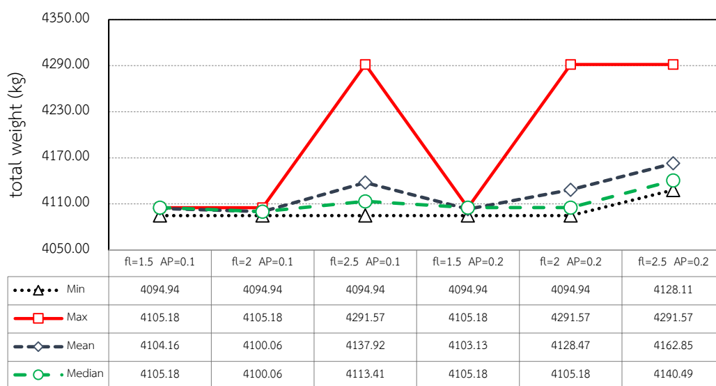
ภาพประกอบ 21 ผลการทดสอบค่าพารามิเตอร์ที่เหมาะสมของ CSA สำหรับโครงข้อหมุน
