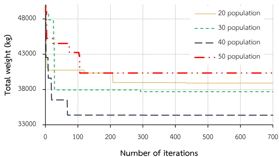
ภาพประกอบ 39 ลักษณะของการหาคำตอบที่เหมาะสมของ WOA สำหรับตัวอย่างที่ 2 โครงข้อ แข็ง 1 ช่วง 10 ชั้น
