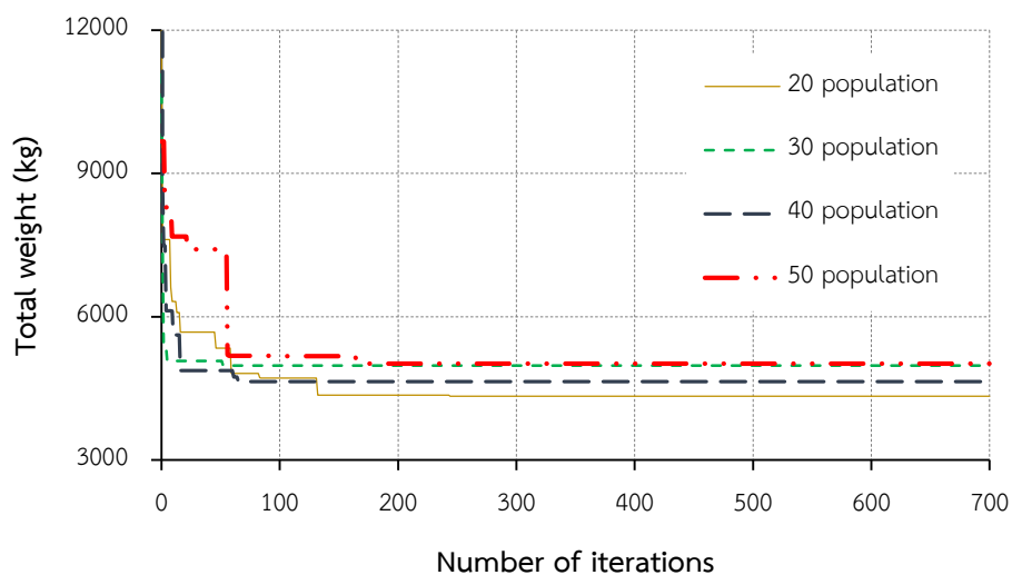
ภาพประกอบ 40 ลักษณะของการหาคำตอบที่เหมาะสมของ WOA สำหรับตัวอย่างที่ 3 โครงข้อ หมุน 10 ชิ้นส่วน โดยใช้หน้าตัดท่อสี่เหลี่ยม
