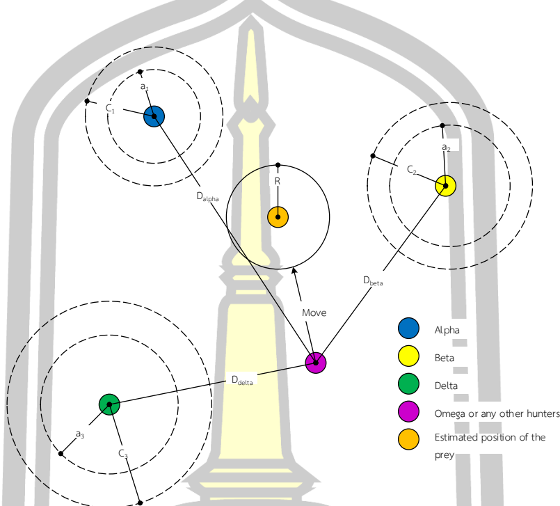
ภาพประกอบ 8 การปรับปรุงตำแหน่งของหมาป่าสีเทา
