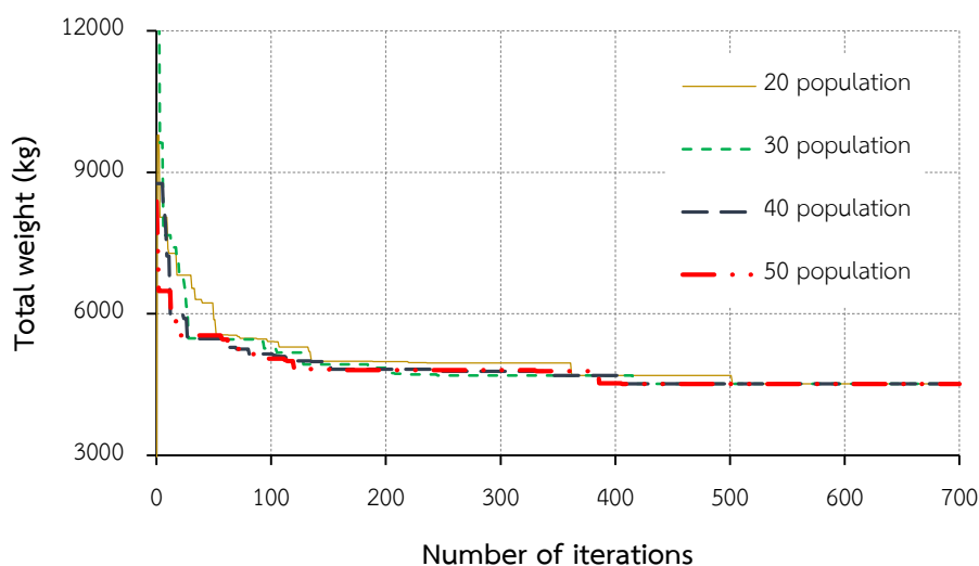
ภาพประกอบ 27 ลักษณะของการรู้เข้าหาคำตอบที่เหมาะสมของ CSA สำหรับตัวอย่างที่ 4 โครงข้อหมุน 18 ชิ้นส่วน โดยใช้หน้าตัดท่อสี่เหลี่ยม
