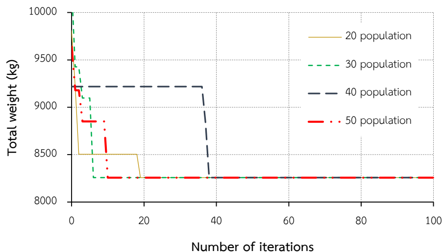
ภาพประกอบ 38 ลักษณะของการหาคำตอบที่เหมาะสมของ WOA สำหรับตัวอย่างที่ 1 โครงข้อ แข็ง 2 ช่วง 3 ชั้น
