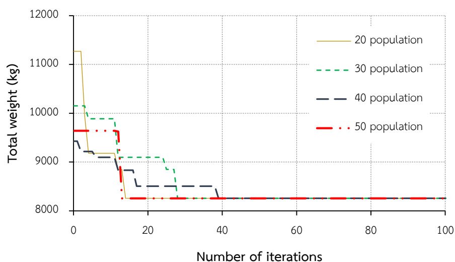
ภาพประกอบ 22 ลักษณะของการลู่เข้าหาคำตอบที่เหมาะสมของ CSA สำหรับตัวอย่างที่ 1 โครงข้อ แข็ง 2 ช่วง 3 ชั้น
